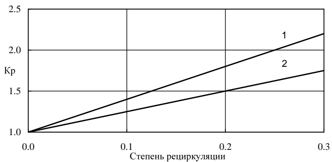
Рисунок Е2 – Зависимость K_p от степени рециркуляции 1 – в дутьевой воздух или кольцевой канал вокруг горелок 2 – в щели под горелками
