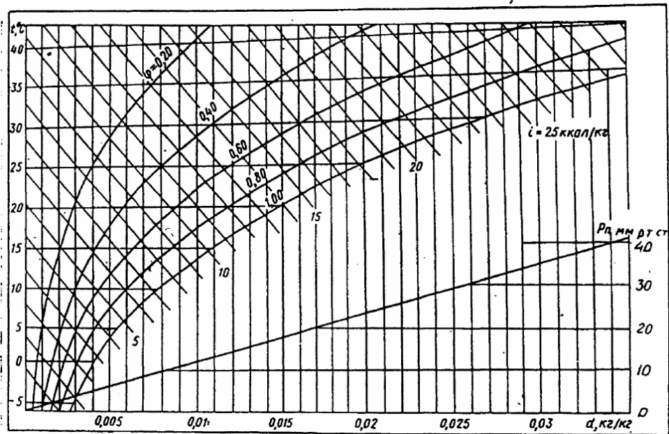
Рис. 1. Диаграмма характеристик влажного воздуха при нормальном атмосферном давлении.
