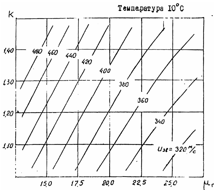
Рис. 2. Скорость звука в сжигаемой смеси
