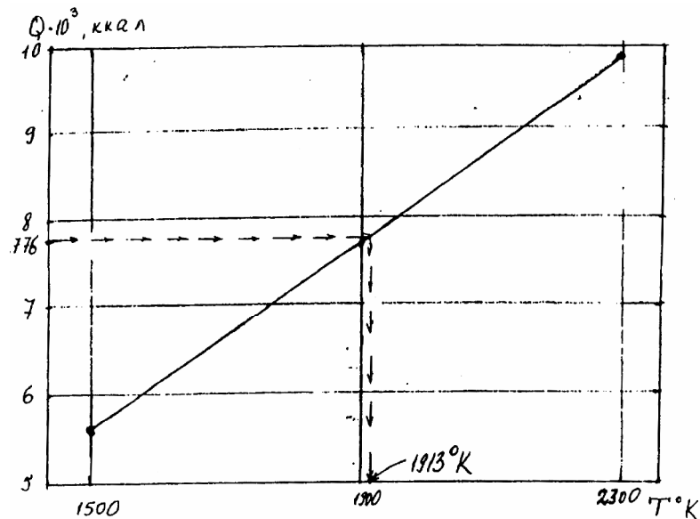
Рис. 6 Пример графического определения температуры продуктов сгорания /попутный нефтяной газ Южно-Сургутского месторождения/.
